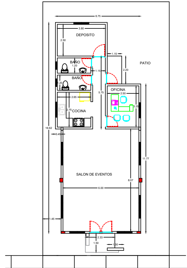
PLANTA DIMENSIONADA
