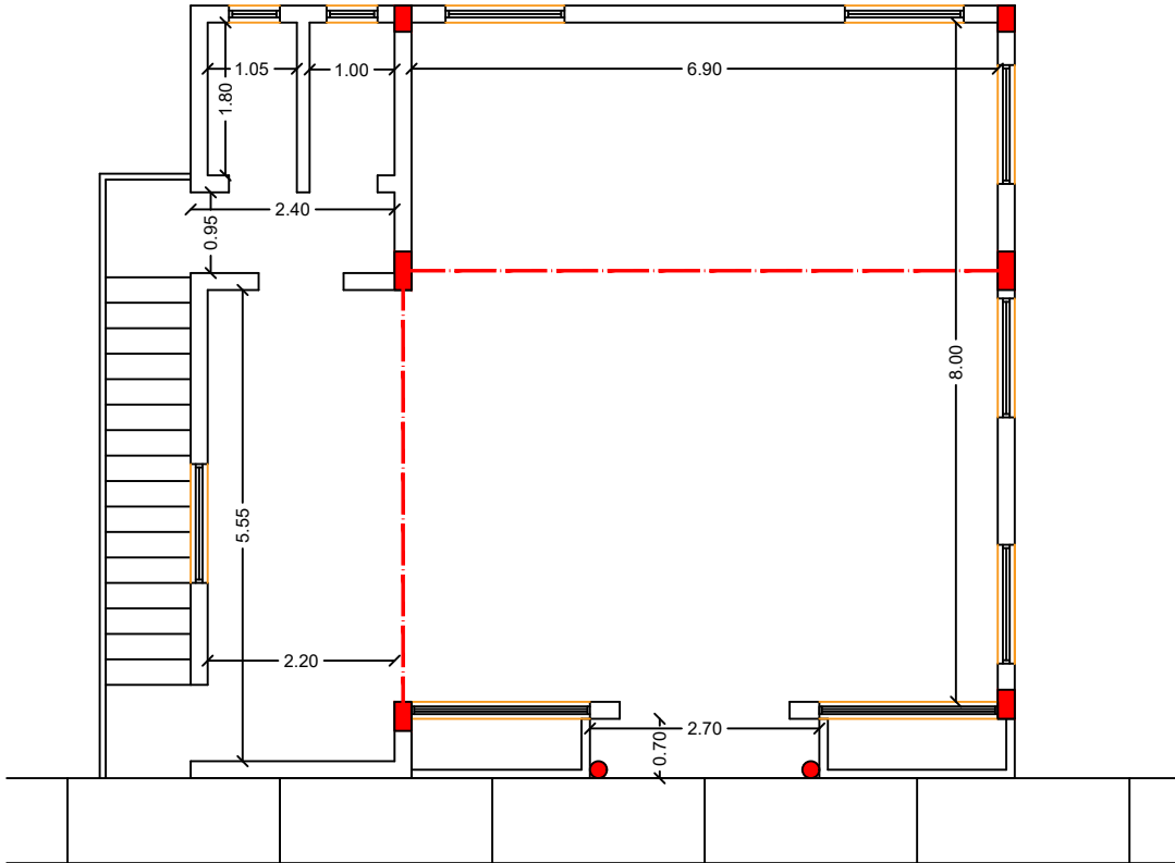
PLANTA ARQUITECTÓNICA 1er NIVEL
