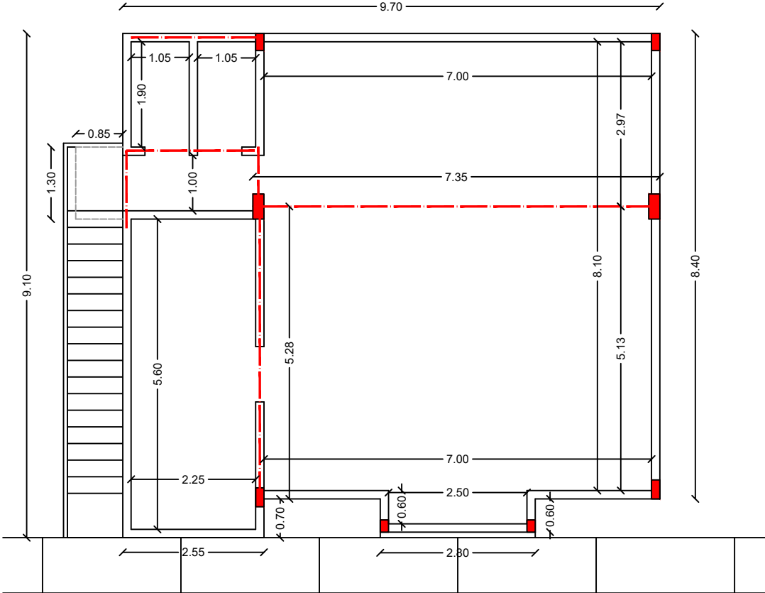
CENTRO COMUNAL PUEBLO NUEVO PLANTA ARQUITECTÓNICA 2do NIVEL
